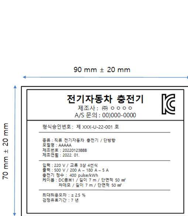
그림 D-1 고정형 충전기 명판 예시
