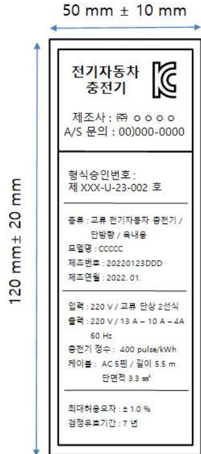
그림 D-2 이동형 충전기 명판 예시
